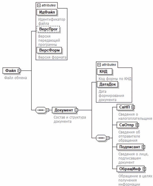
Рисунок 1. Диаграмма структуры файла обмена
