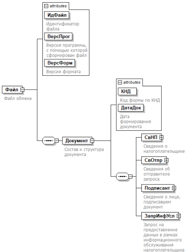
Рисунок 1. Диаграмма структуры файла обмена
