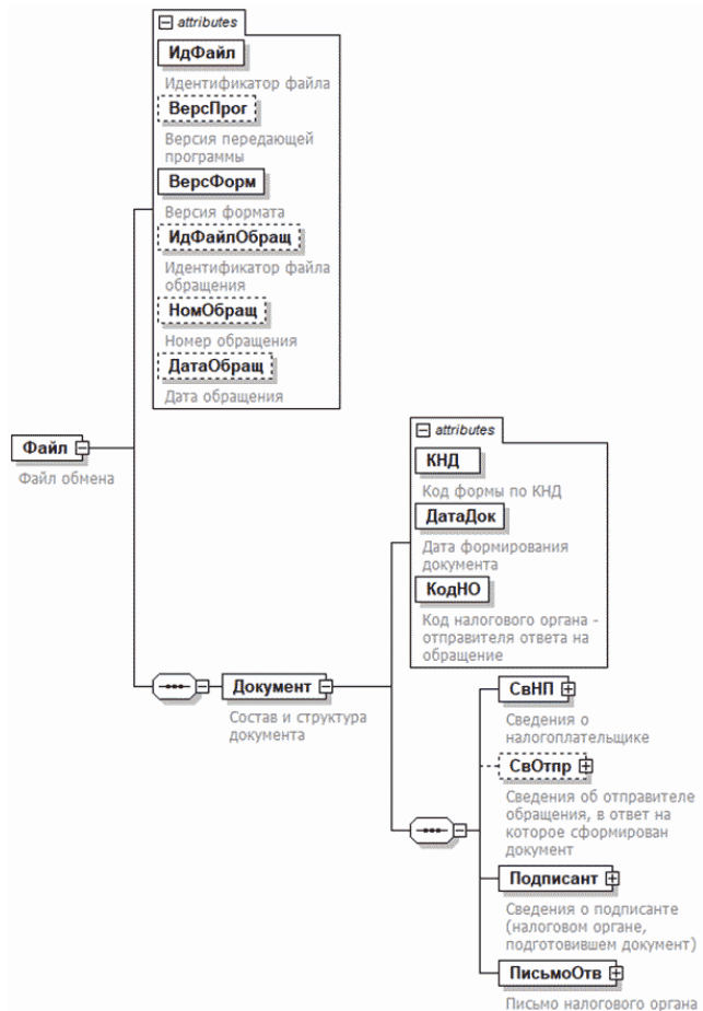
Рисунок 1. Диаграмма структуры файла
